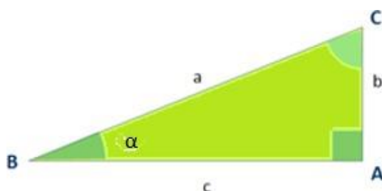
Imagen 6: Triángulo rectángulo
